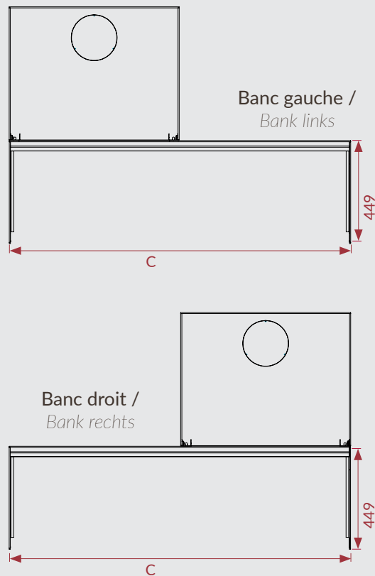
DIMENSIONS / AFMETINGEN
